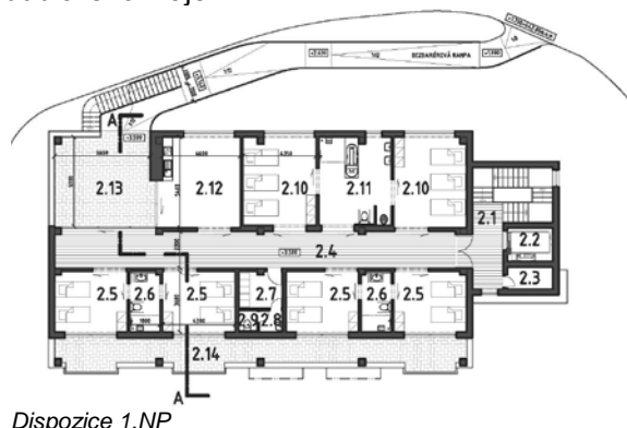
Dispozice 1.NP
