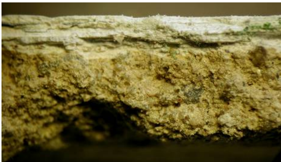
Statigrafie nátěrových a omítkových vrstev. Na snímku souvrství vápenných nátěrů a měkká vápenná omítka (S140/1)
